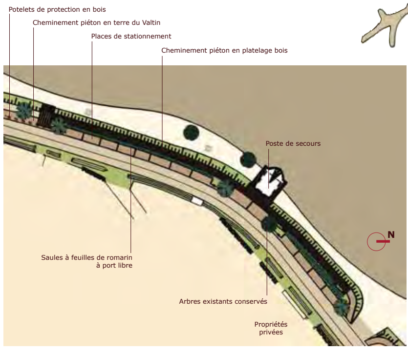
Détail du plan de masse et coupe au niveau du cheminement en platelage, URBAM Conseil
