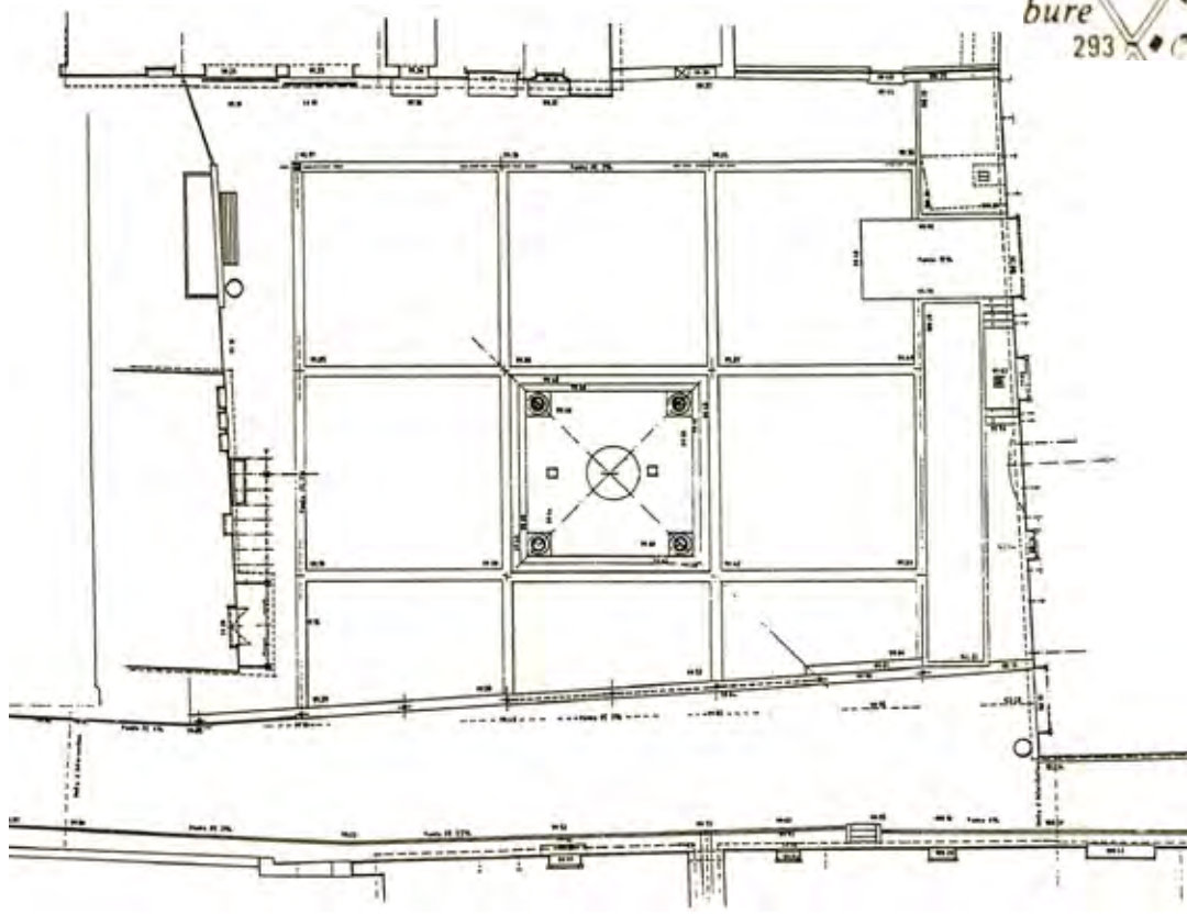
Projet d'aménagement de la place du Puits P. Gosselin, architecte
